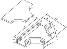
XQJ-C-03A 型水平三通 XQJ-C-03A Horizontal 3-way
