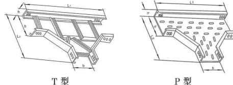
T 型
