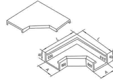
XQJ-C-02A 型水平弯通 XQJ-C-02A Horizontal Curved
